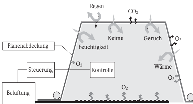
Abb. 1. Verfahrenskomponenten und Prozessabläufe in einer abgedeckten und geregelten Miete.
