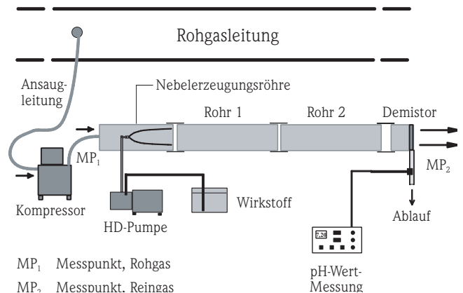
Abb. 1. Schematischer Aufbau des mobilen Mischnebelabsorbers.
