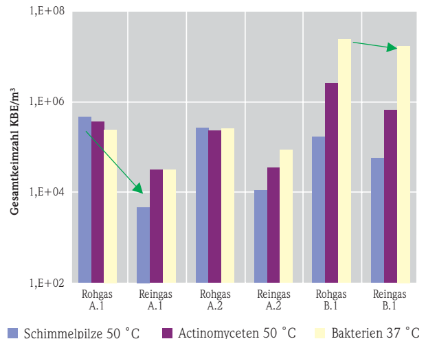
Abb. 3. Bioaerosolemissionen-Biofilter.
