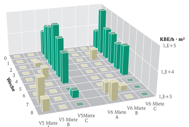
Abb. 9. Flächenspezifische Keimfracht von Aspergillus fumigatus im Zeitverlauf bei zwei Versuchen mit abgedeckten Mieten (A, B) im Vergleich zu einer nicht abgedeckten Miete (C).
