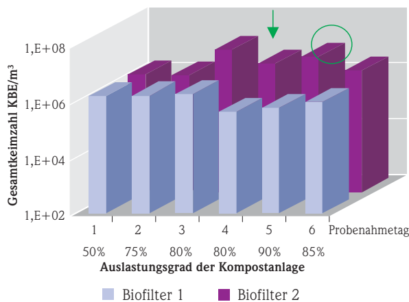
Abb. 2. Biofilter-Optimierung (geschlossene Kompostierungsanlage; Bio- und Grünabfall <math>< 10000 \text{ Mg/a}</math>; Filtermaterial: Siebreste/Rindenmulch ab Probenahmetag 4. Filtermaterial 1 Grünschnitt, Rinden Filtermaterial 2 Kokosfasern)
