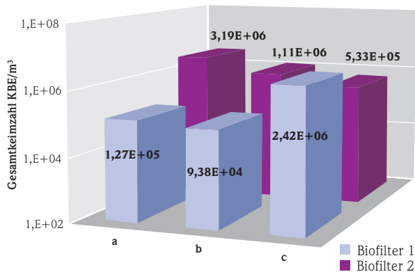
Abb. 1. Messwertstreuung (gefasste Abluftquelle, Biofilter <math>< 1000 \text{ m}^3/\text{h}</math>).
