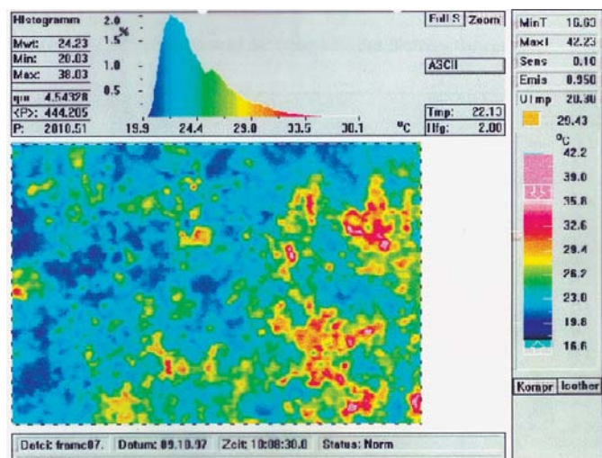
Abb. 5. Biofilter 3 mit gleichmäßiger Rohgastdurchströmung.
