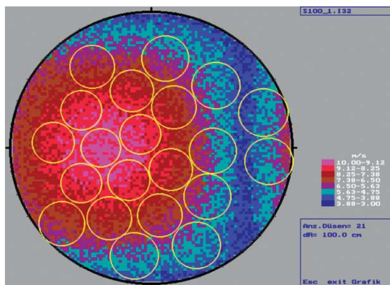
Abb. 2. Berechnete Platzierung von Düsen in einem Strömungsfeld bekannter Strömungsgeschwindigkeit.
