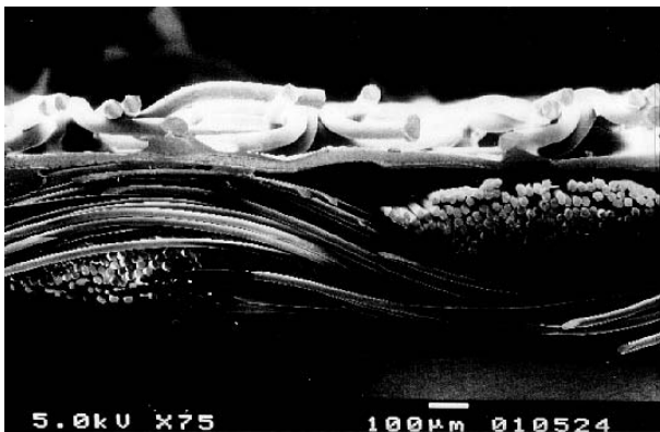
Abb. 3. Elektronenmikroskopische Aufnahme eines Querschnittes durch ein Textillaminat.
