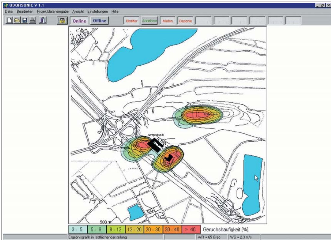
Abb. 3. Geruchsfahne bei labiler Schichtung der Atmosphäre.
