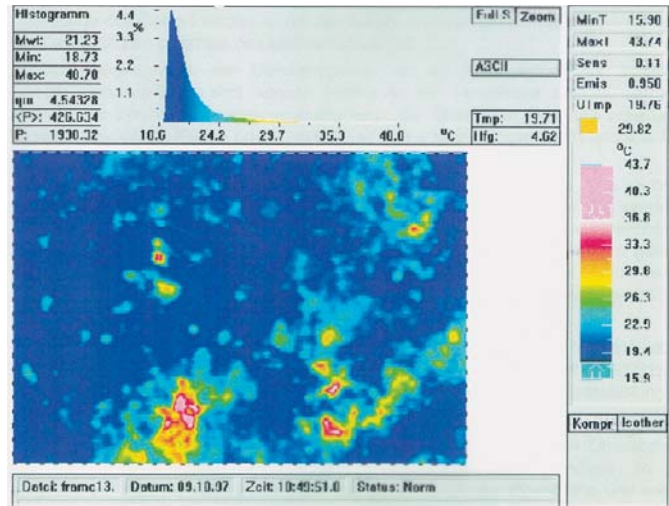
Abb. 3. Biofilter 1 mit großen Bereichen geringer Durchströmung.
