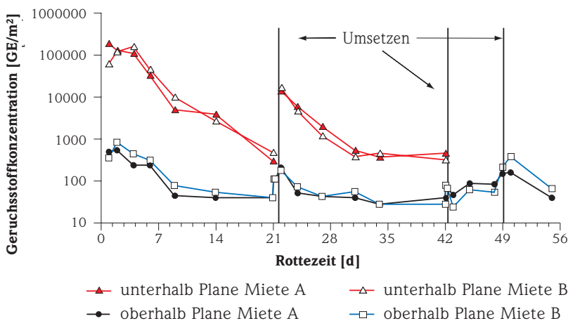
Abb. 6. Geruchsstoffkonzentrationen der abgedeckten Miete A und Miete B oberhalb und unterhalb der Abdeckung im Rotteverlauf (Methode C 30 , Versuch 5).
