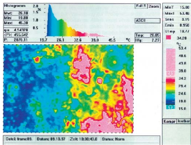
Abb. 4. Biofilter 2 mit großen Inhomogenitäten der Temperaturverteilung.
