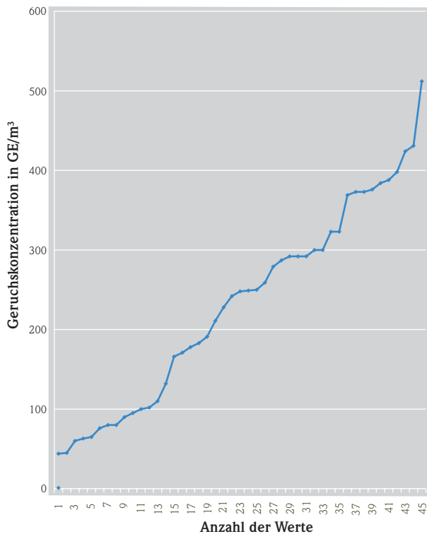
Abb. 1. Häufigkeitsverteilung Reingaskonzentration Biofilter (HLUG).
