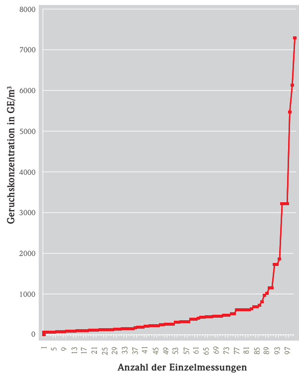
Abb. 2. Häufigkeitsverteilung Reingaskonzentration Biofilter (TÜV).
