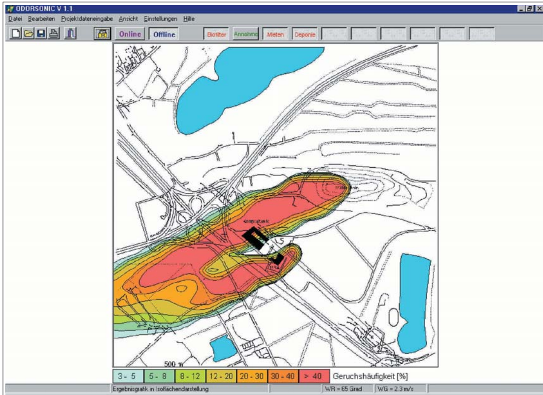
Abb. 2. Geruchsfahne bei stabiler Schichtung der Atmosphäre.
