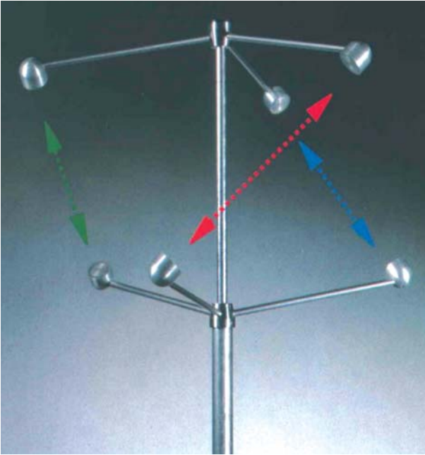
Abb. 1. Ultraschallanemometer zur Ermittlung der vertikalen und horizontalen Austauschparameter.
