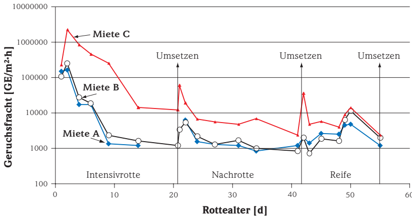
Abb. 7. Auswirkungen des Einsatzes von Planenabdeckungen bei Miete A und Miete B auf die Geruchsemissionen im Rotteverlauf (Methode C 30 , Versuch 6).
